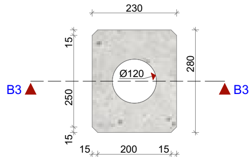
PELARE BETONG 1:10
