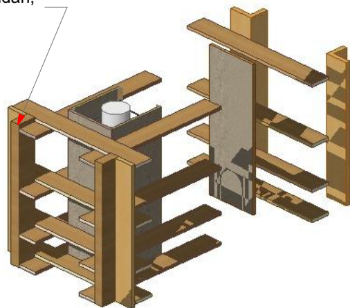
FORMBYGGNAD 3D 1:200
