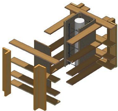
FORMBYGGNAD 3D 1:200
