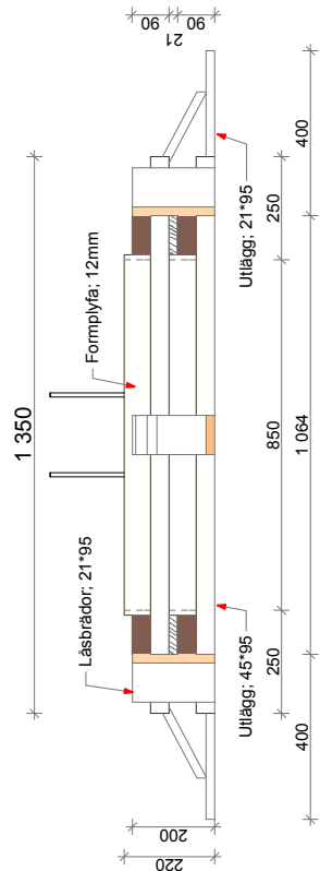
B1 SEKTION KORTSIDA 1:20
