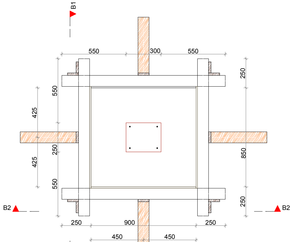
PLAN 1:20
