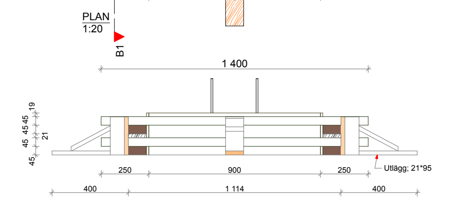
B2 SEKTION LÅNGSIDA 1:20
