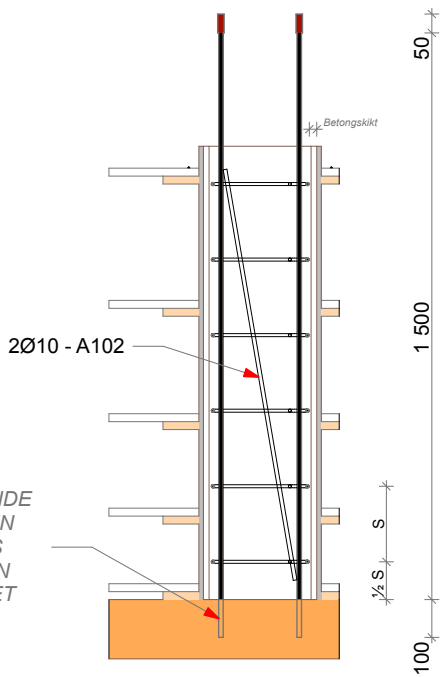
B4 SNITT PELARE ARMERING 1:20
