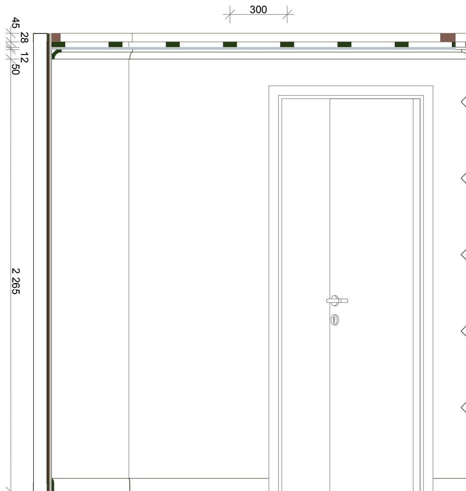
A5 Snitt genom taket 1:20
