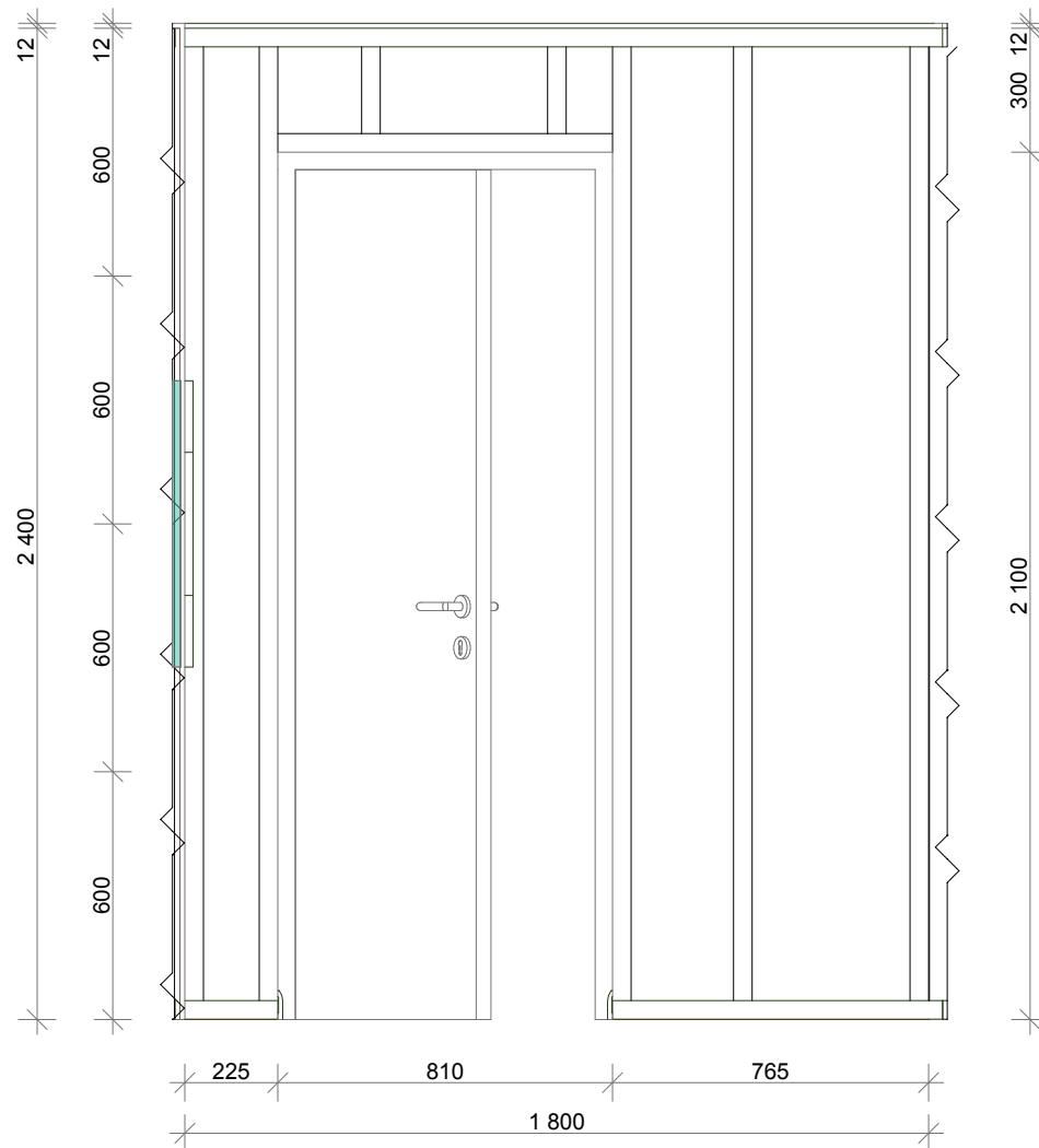
A2 - SEKTION 1:20
