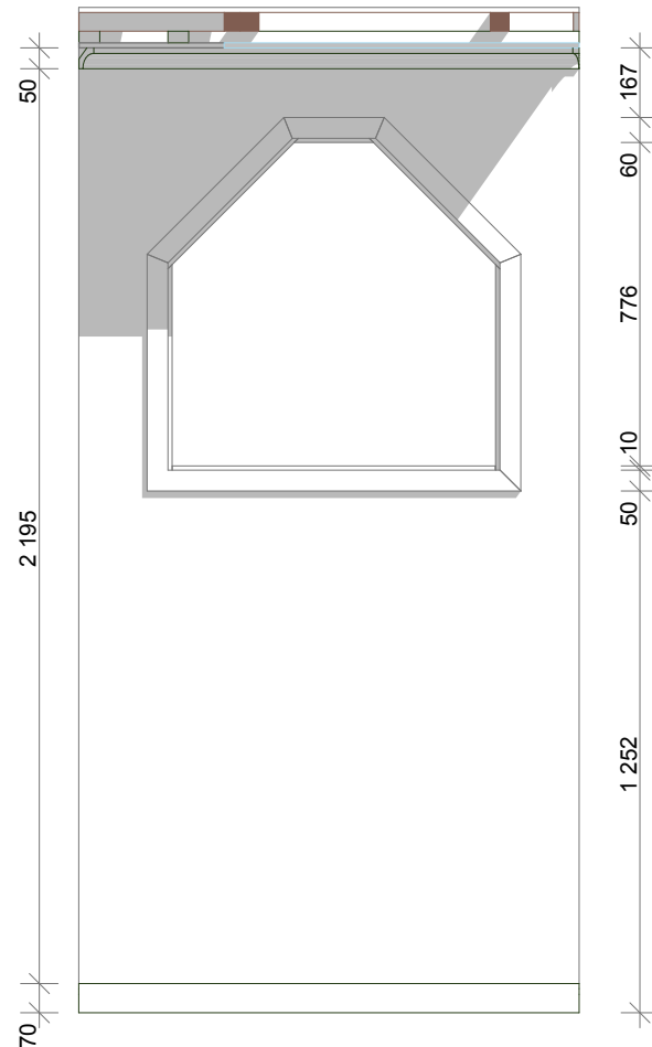
B2 - ELEVATION 1:20
