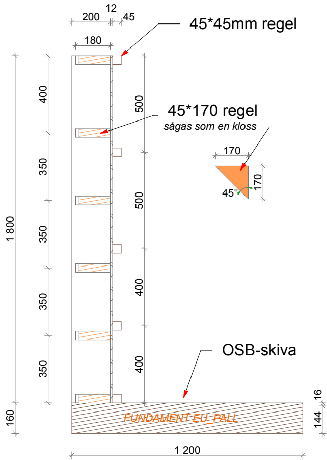
VÄGG AVSTÄNGARE o FUNDAMENT 1:20
