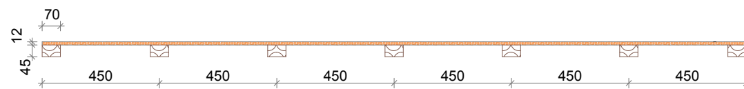
F5 SEKTION gm FUNDAMENT (1) 1:20
