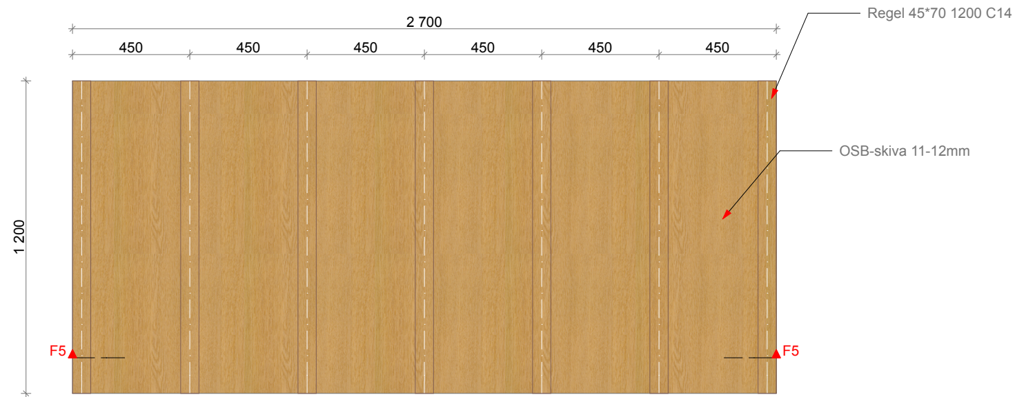
FUNDAMENT-TÄVLINGSYTA (1) 1:20
