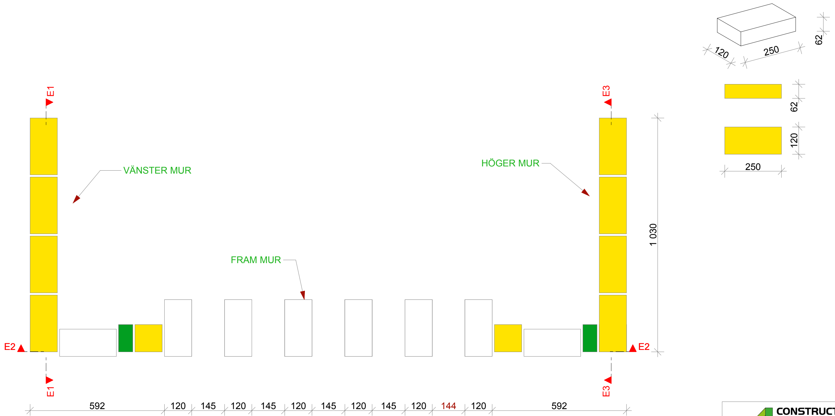
1. PLAN 1 ETT SKIFT 1:10
