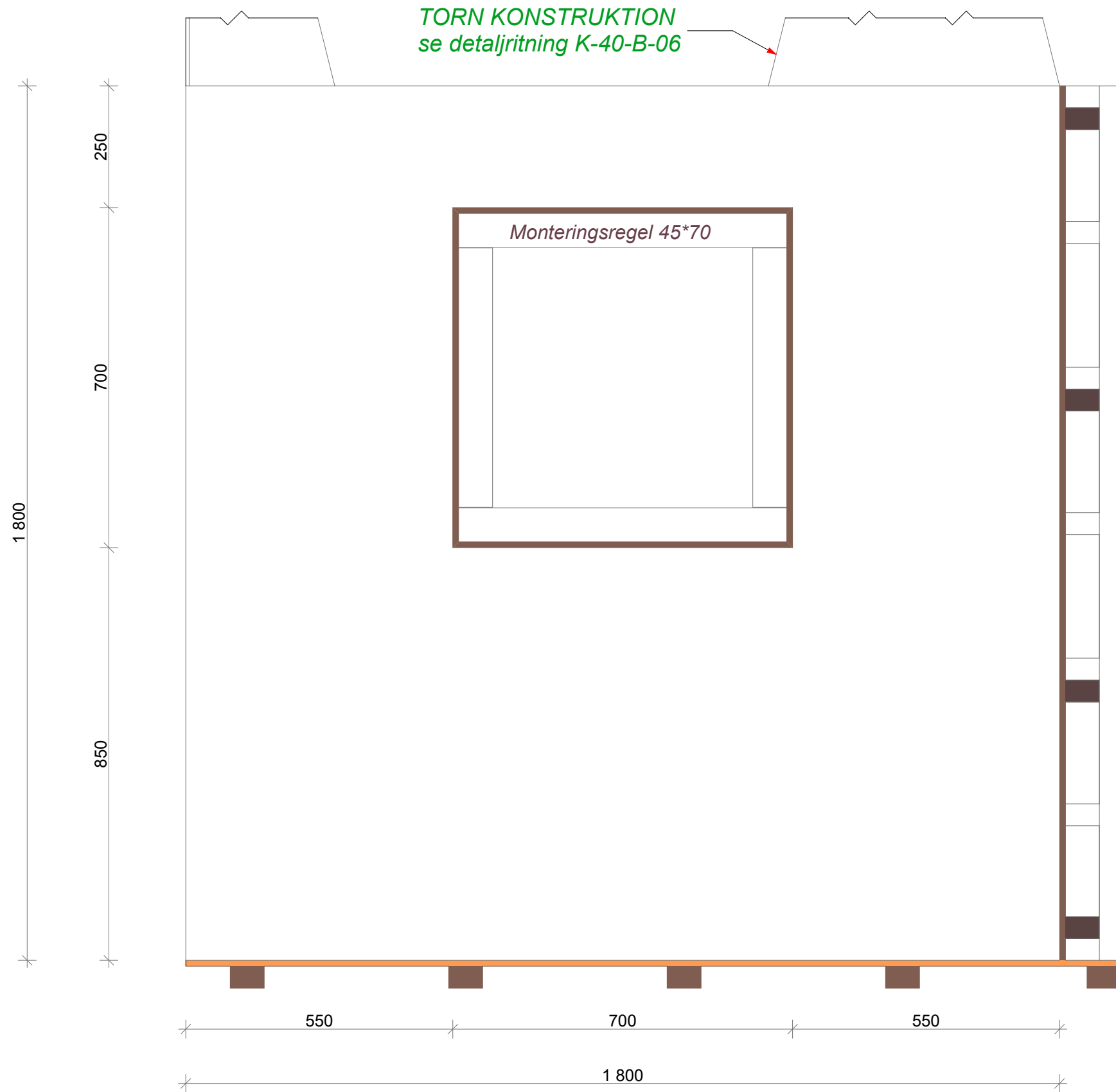
F2 ELEVATION V-1800 (1) 1:10
