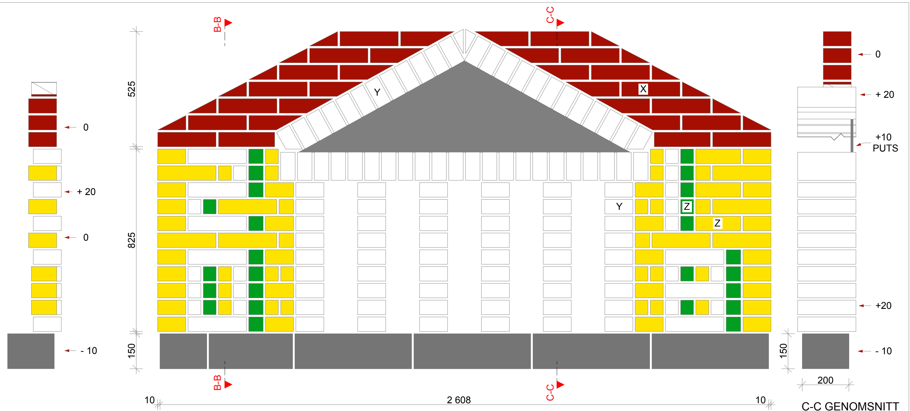
B-B GENOMSnitt V.SIDA FRONT 1:10
